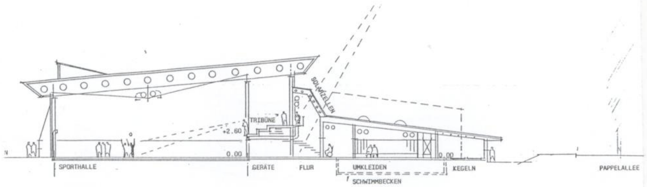
NORD-SÜD-SCHNITT M 1:200
